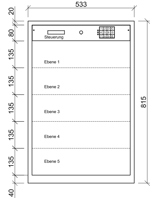
Gehäuse B 5 H/B/T 815/533/580mm
