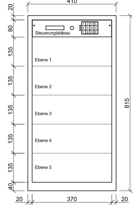
Gehäuse A 5 H/B/T 815/410/580mm
